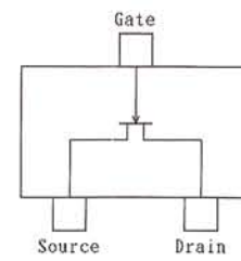
2SK160 (K5) (Q6510, 6511)
