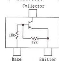
FN1A4P (M34) (Q3031, 3032, 3033 3034)
