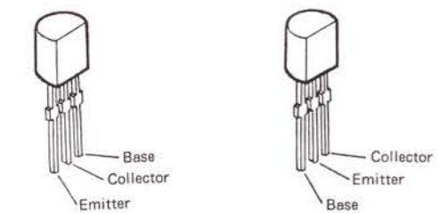
2SC2026 (Q1008) 2SD667C (Q1101) 2SA1283D (Q1053, 1054)
