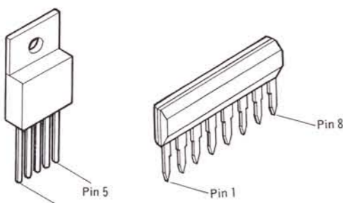
TDA2003H (Q1034) M5223L (Q1065, 1068, 1082, 1088, 1094)
